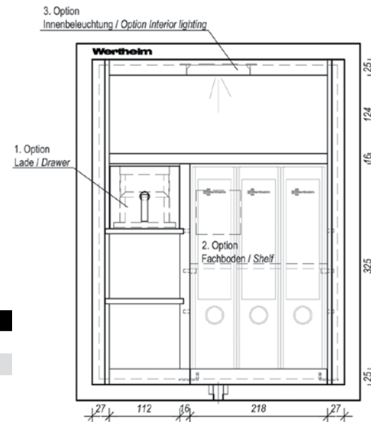
Ansicht aus Zeichnung ALZ 007 200
