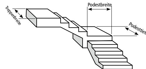
5. Treppe 90° abgewinkelt mit Podest
