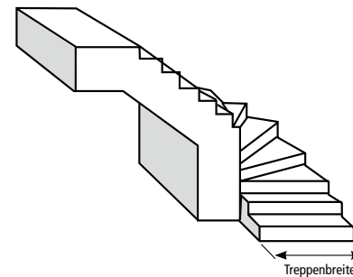
3. Treppe mit einem 90° Wendepunkt
